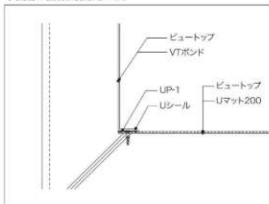
平面部：機械的固定工法
