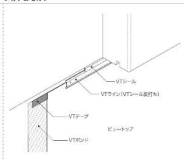
水切り目地有り
