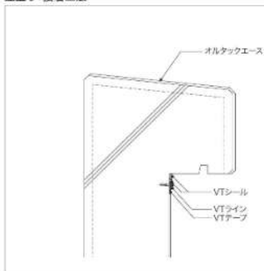
立上り：接着工法
