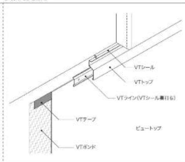
水切り目地無し
