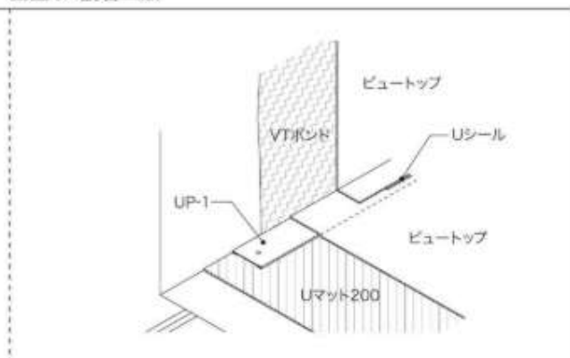
立上り：接着工法
