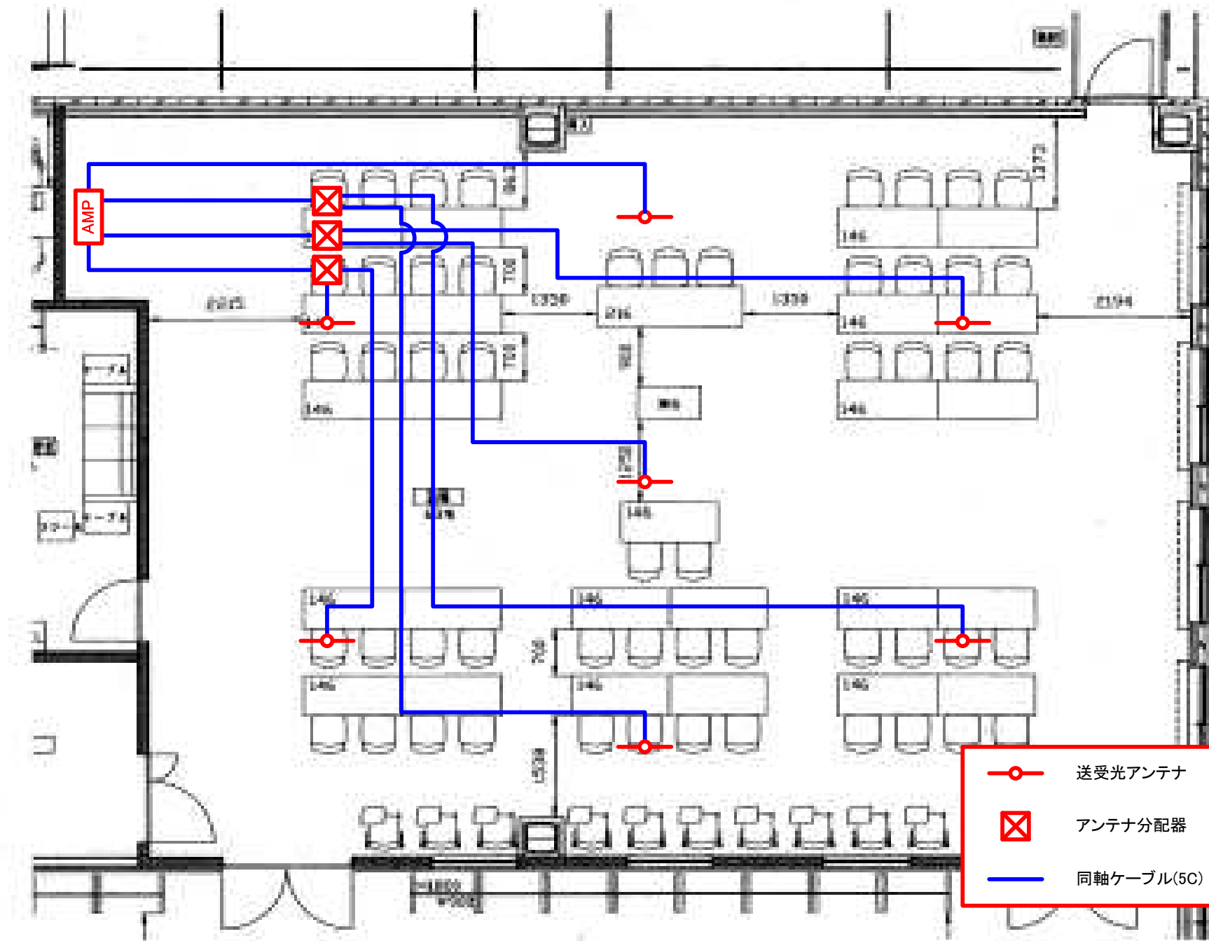
(別紙1) 赤外線送受光アンテナ配置図
